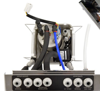
SATURAČNÍ SUD
